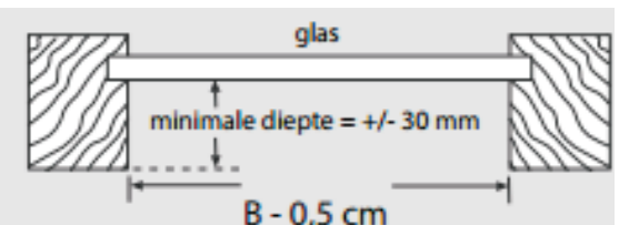
Afb. 2 kozijn met rechte glaslat
